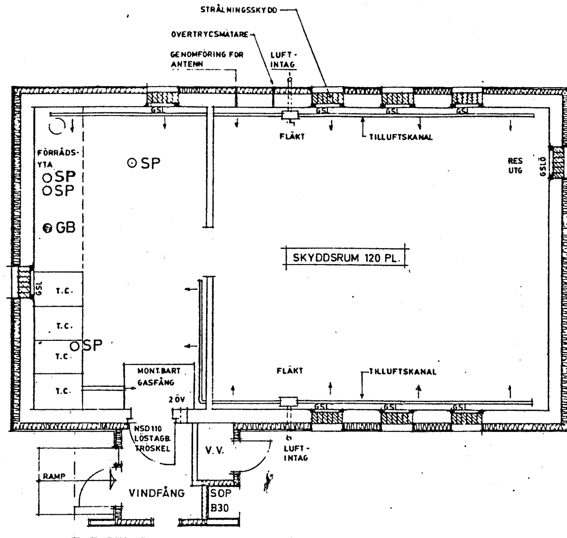
PLAN SKYDDSRUM
